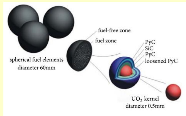
TRISO paliva pro bloky HTR-PM
