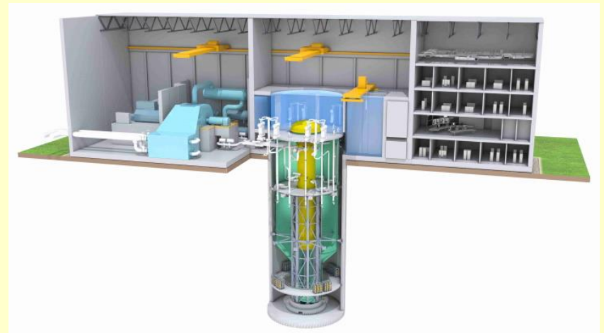
Schéma reaktoru BWRX-300
